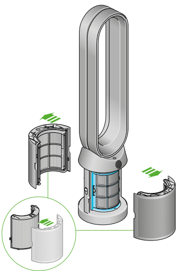
二合一空氣清淨機濾網蓋打開，顯示位於濾網蓋的二合一 HEPA+活性碳濾網。箭頭顯示活性碳濾網直接安裝到機器底座，且濾網蓋需組裝到機器底座上。
