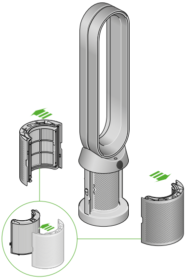
二合一空氣清淨機濾網蓋打開，顯示位於濾網蓋的二合一 HEPA+ 活性碳濾網。 箭頭顯示濾網蓋需組裝到機器底座上。
