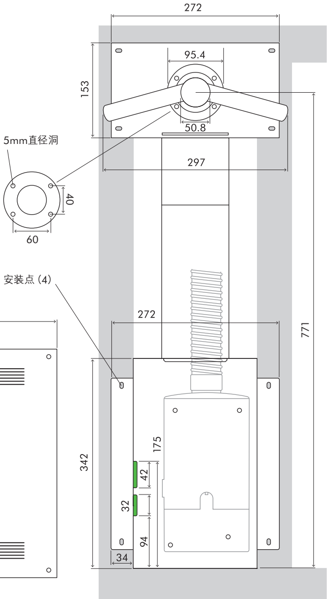
前端视图
