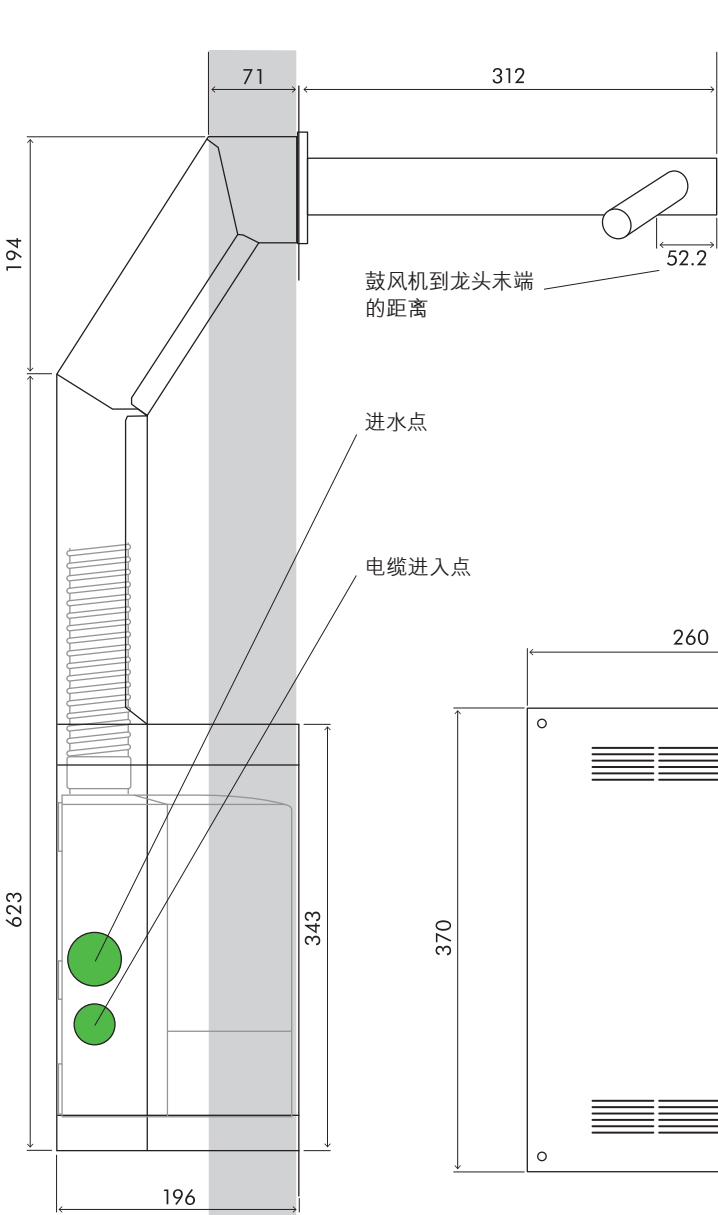
旁视图
