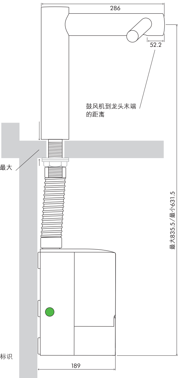
旁视图
